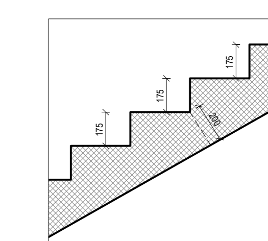
Detaji D4 Shkalla 1 : 20
