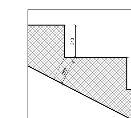
Detaji D2 Shkalla 1 : 20
