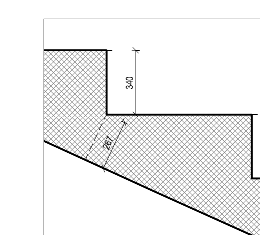
Detaji D1 Shkalla 1 : 20
